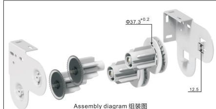
ZFADA38B Roller blind mechanism ADA 38B 3800控制器 (不含支架)
